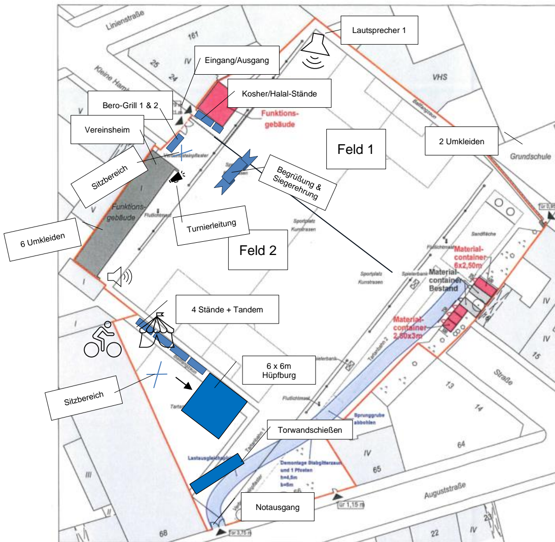
Baustelleneinrichtungsplan M 1:500
